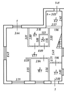
План 1 этажа
