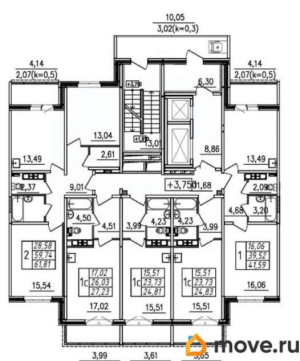
ПЛАН ТИПОВОГО ЭТАЖА СЕКЦИЯ 5
