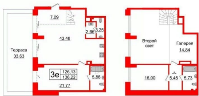
План 1 уровня h=2,70 м
