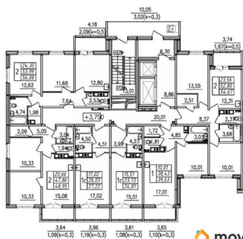
секция 1 ПЛАН ТИПОВОГО ЭТАЖА
