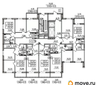
секция I ПЛАН ТИПОВОГО ЭТАЖА
