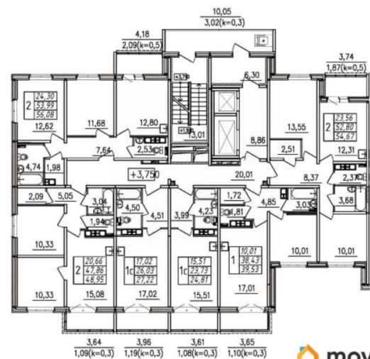
секция 1 ПЛАН ТИПОВОГО ЭТАЖА
