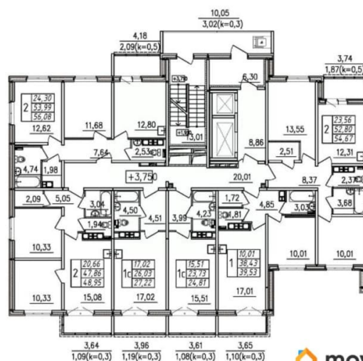
секция 1 ПЛАН ТИПОВОГО ЭТАЖА
