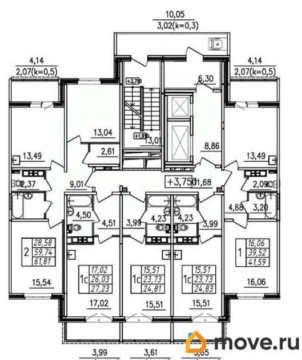
ПЛАН ТИПОВОГО ЭТАЖА СЕКЦИИ 5
