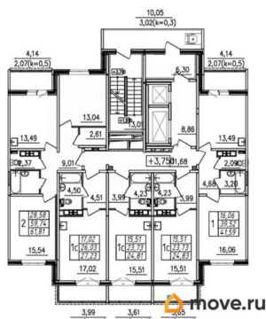
ПЛАН ТИПОВОГО ЭТАЖА СЕКЦИИ 5
