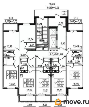
ПЛАН ТИПОВОГО ЭТАЖА СЕКЦИЯ 2
