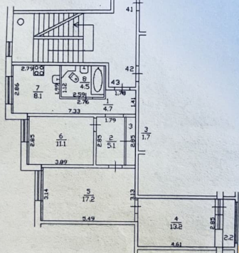
План части 3-го этажа 3 подъезд
