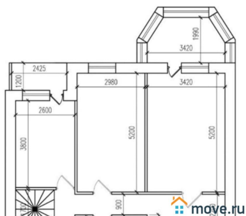
План 2 этажа
