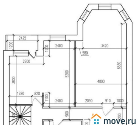
План 1 этажа
