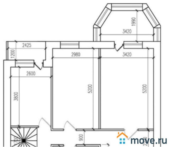
План 2 этажа
