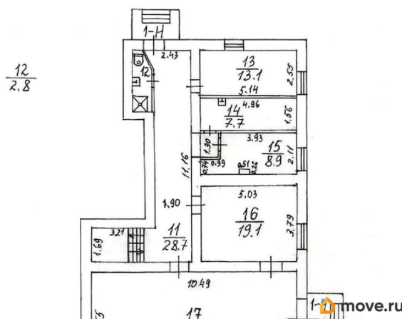
План 1 этажа
