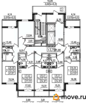
ПЛАН ТИПОВОГО ЭТАЖА СЕКЦИЯ 5
