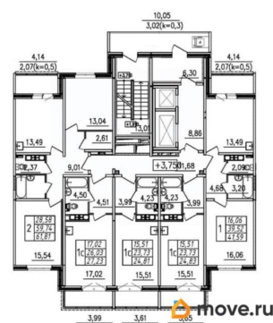
ПЛАН ТИПОВОГО ЭТАЖА СЕКЦИЯ 2
