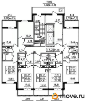
ПЛАН ТИПОВОГО ЭТАЖА СЕКЦИЯ 4
