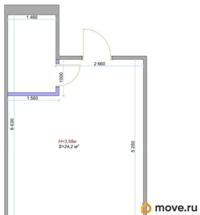
План возведения перегородок
