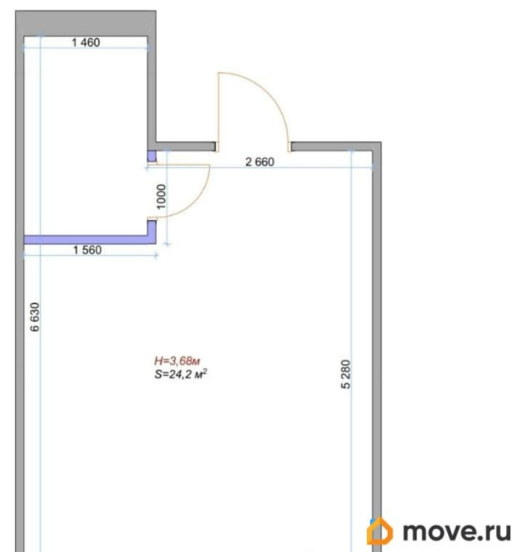
План возведения перегородок
