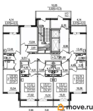
ПЛАН ТИПОВОГО ЭТАЖА СЕКЦИЯ 2
