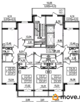
ПЛАН ТИПОВОГО ЭТАЖА СЕКЦИЯ 2
