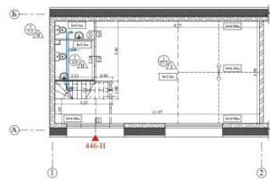
План помещений нежилого помещения после перепланировки
