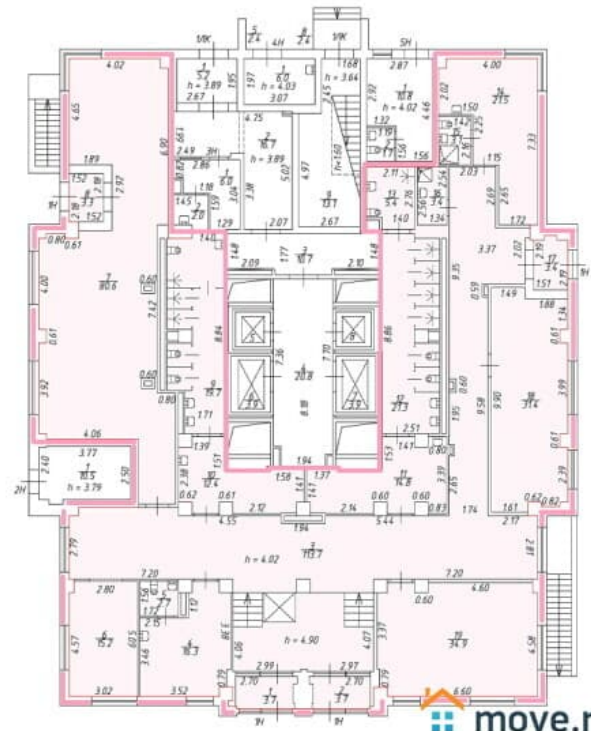
План 1 этажа
