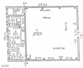
План 1 этажа
