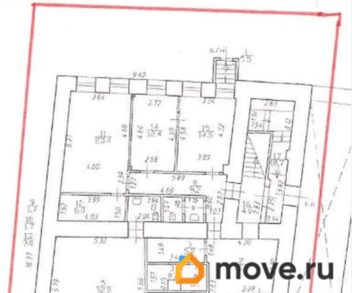
План 2го этажа. S=331 кв.м.
