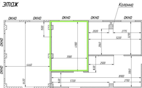
2-ой этаж
