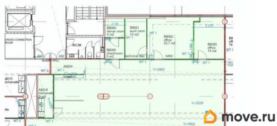
8 этаж, Секция А, планировка офиса
