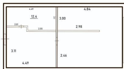
План помещения 4317 3 этаж
