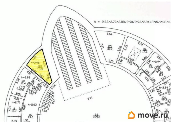
Вестибюль ст.м. «Проспект Большевиков» (1 подземный этаж)
