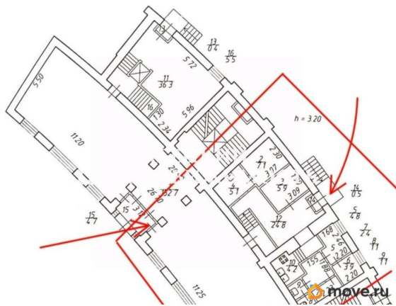
План 1 этажа
