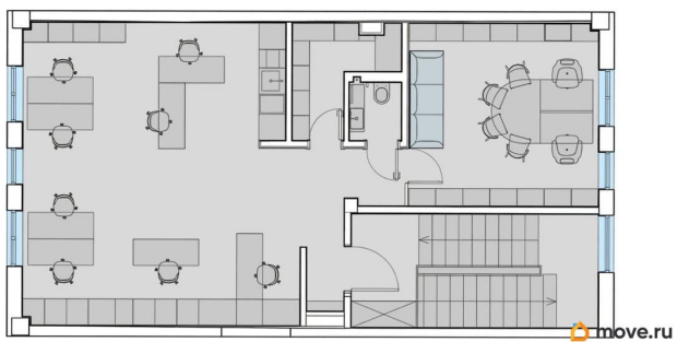
2 ЭТАЖ
