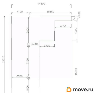
Рис. 2 - план помещения с линейными размерами (пр. Испытателей, д.37, 1-й этаж) S = 174 кв.м.
