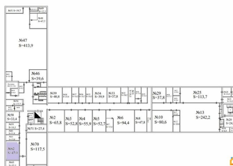
Литера "А" План 2 этажа
