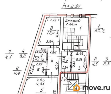
План 1 этажа
