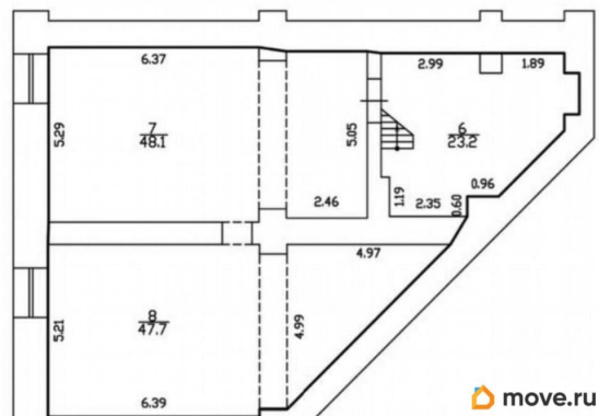
План части подвала
